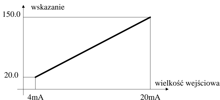
Rys. 4. Przykładowy przebieg "rosnącej" charakterystyki wejściowej regulatora
