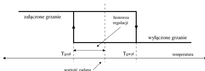
Rys. 2. Algorytm pracy regulatora ST-54A
