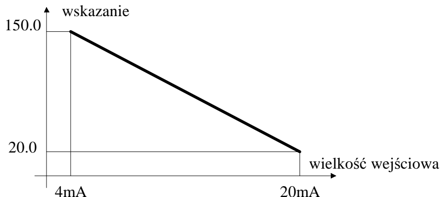
Rys. 5. Przykładowy przebieg "opadającej" charakterystyki wejściowej regulatora
